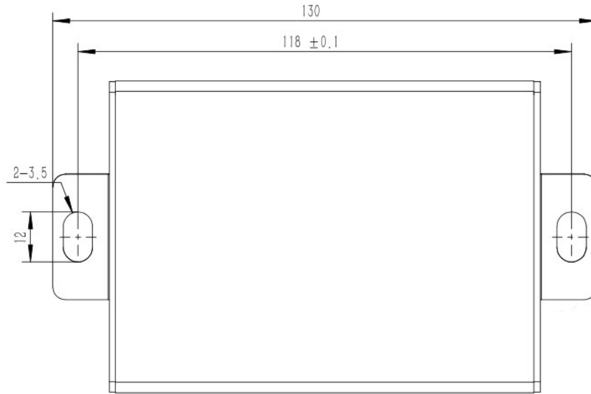
顶视图
