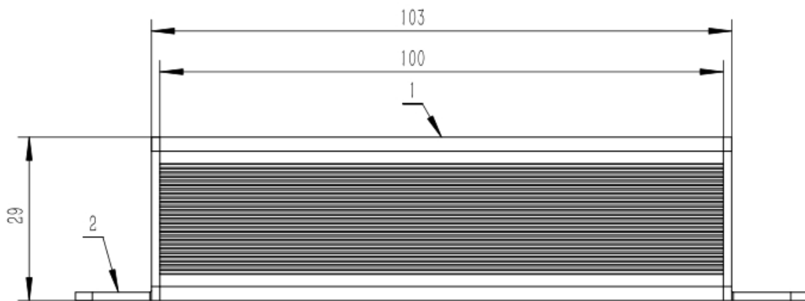
侧视图
